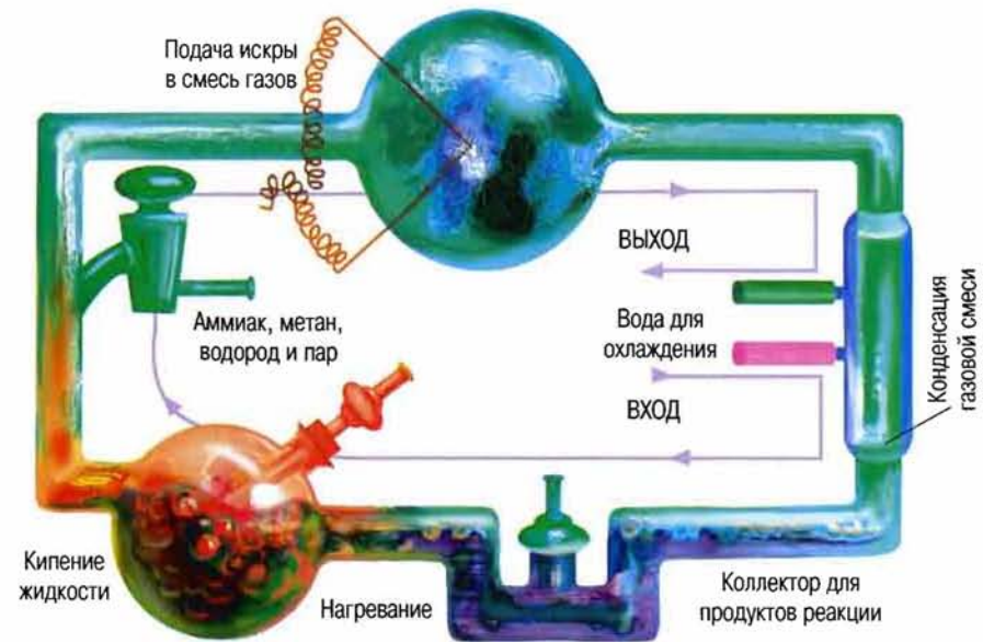
Опыт Миллера
