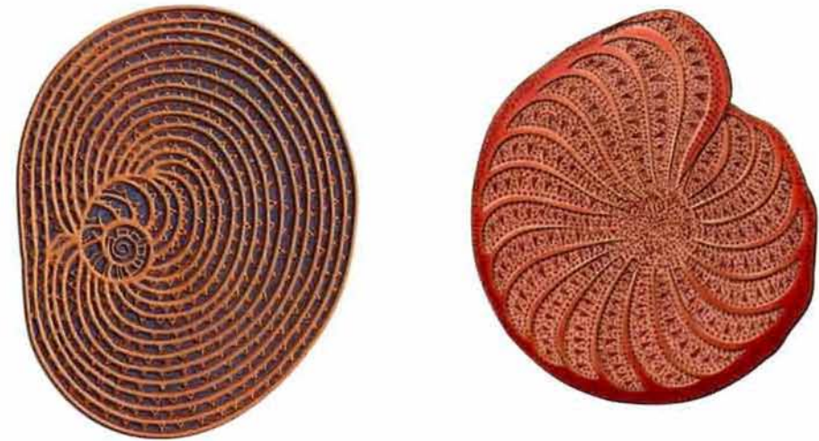
Раковины фораминифер
