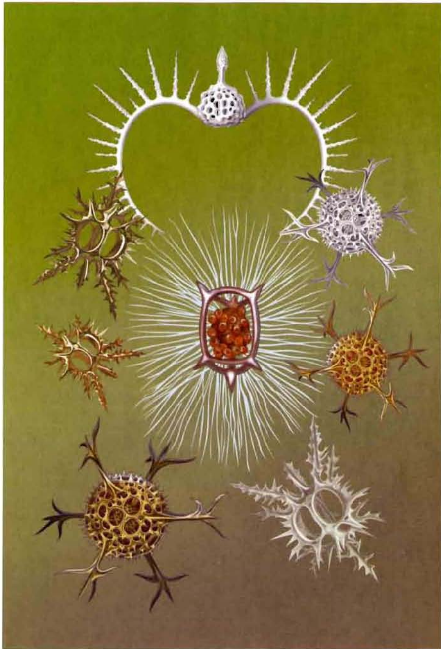
Радиолярии
