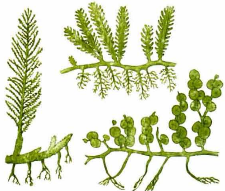
Зеленые водоросли
