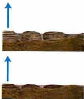
Образование строматолитов
