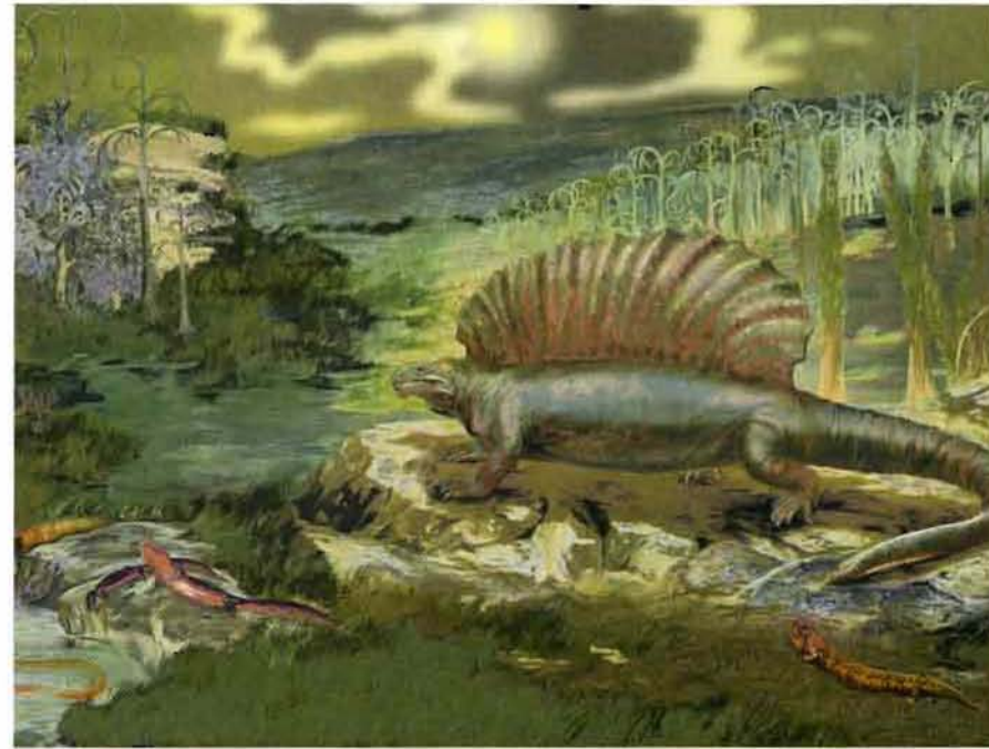
Эдафозавр
